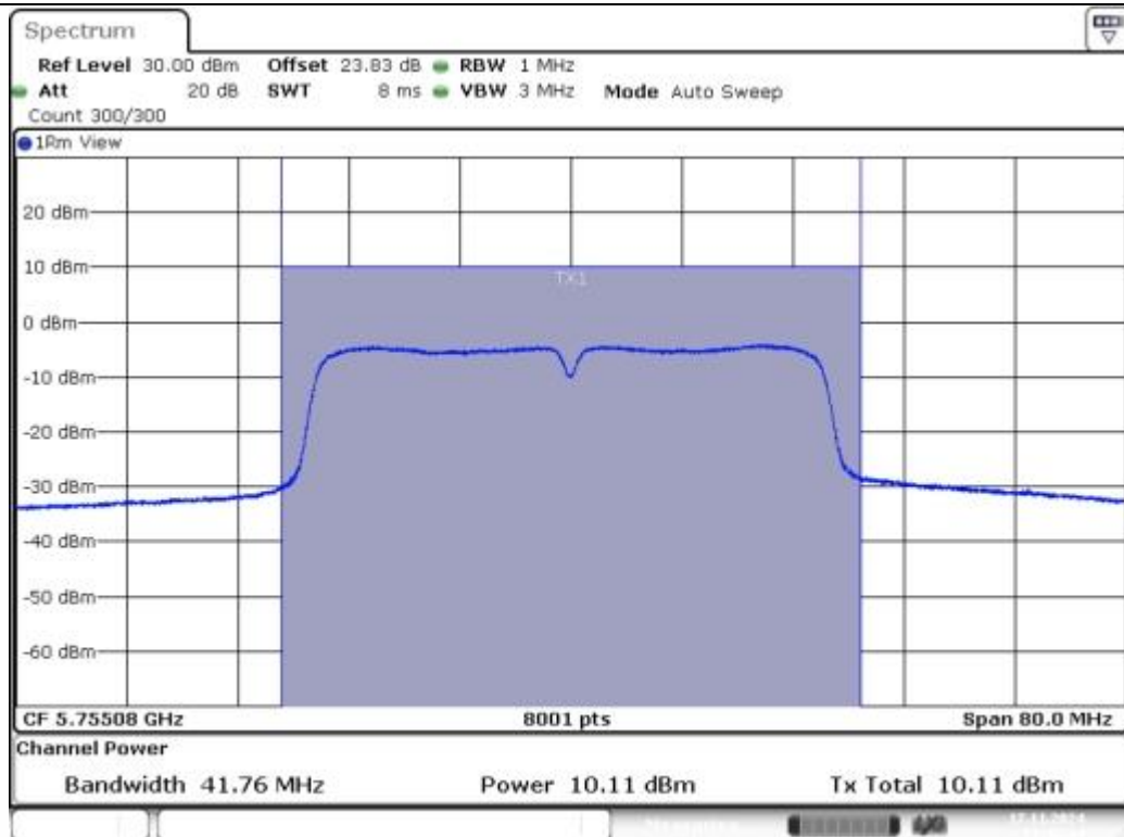
11N40SISO-Ant1-5755-PASS
