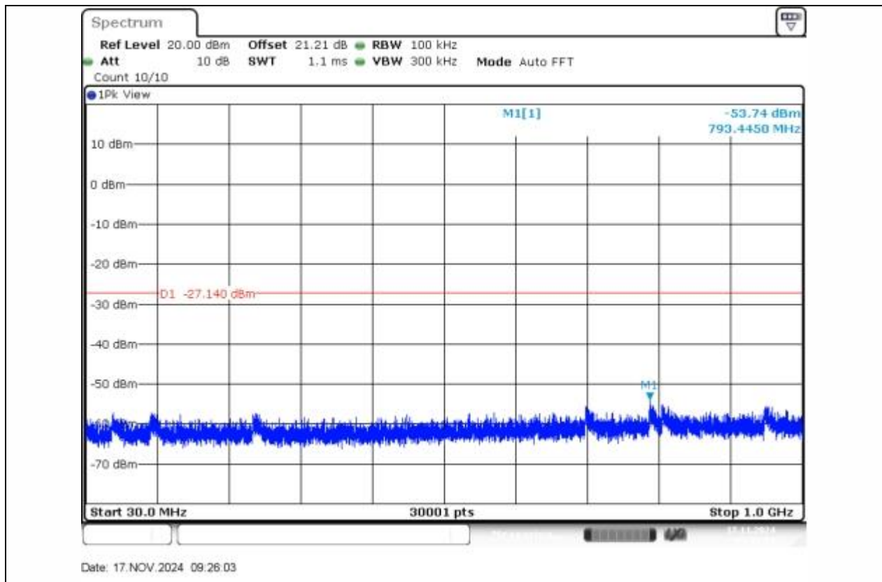
11G-Ant1-2412-30~1000-PASS
