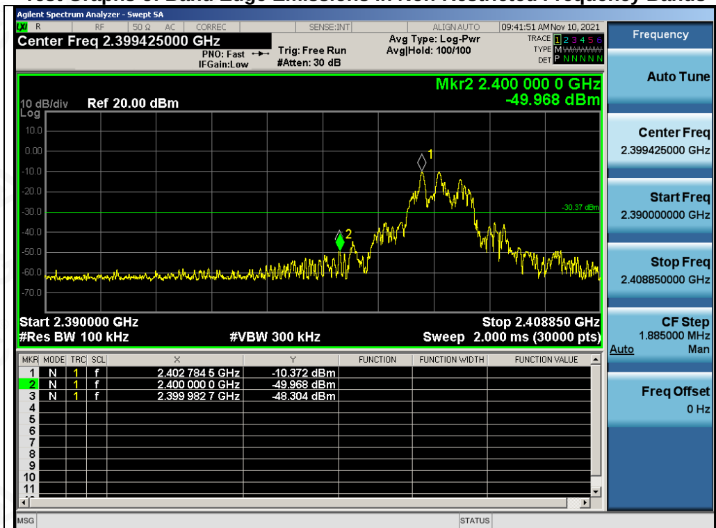
Test_Graph_ANT1_2403.85_Lower Band Edge Emissions
