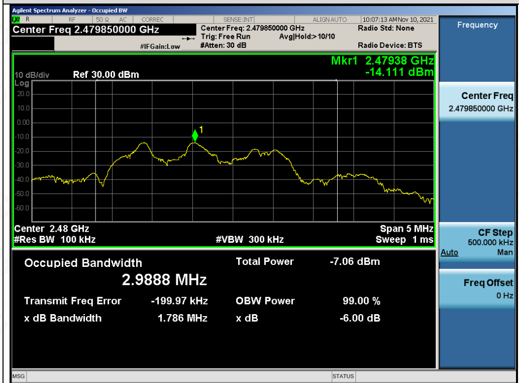
Test_Graph_ANT1_2479.85_DTSBW
