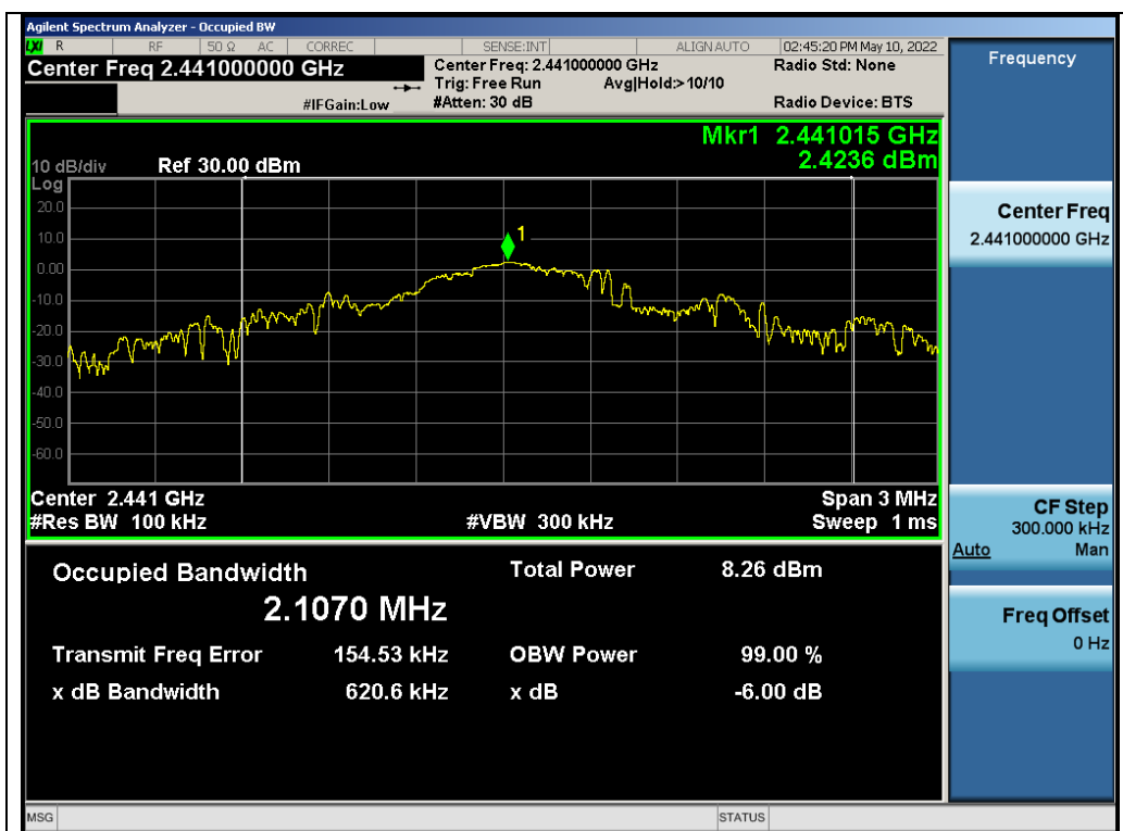
Test_Graph_2.4G_ANT1_2441_DTSBW
