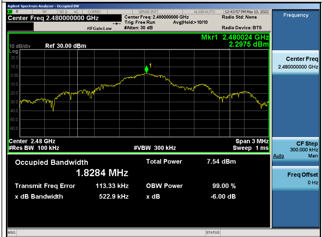
Test_Graph_2.4G_ANT1_2480_DTSBW
