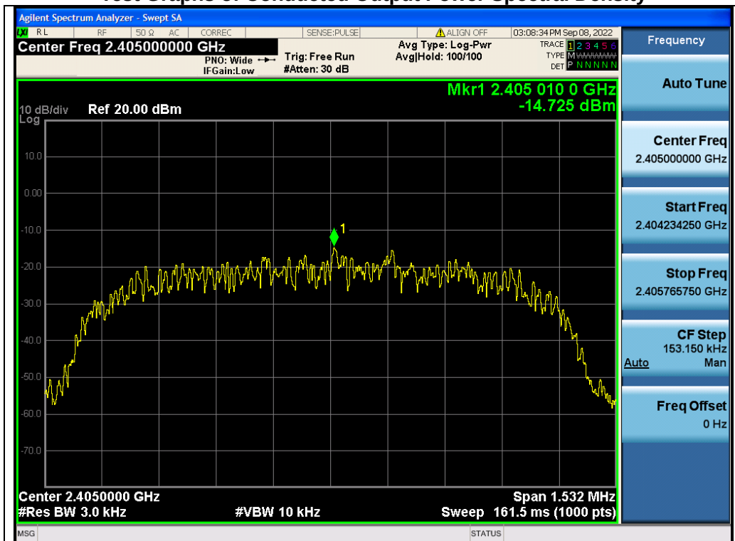
Test_Graph_GFSK_ANT1_2405_PSD
