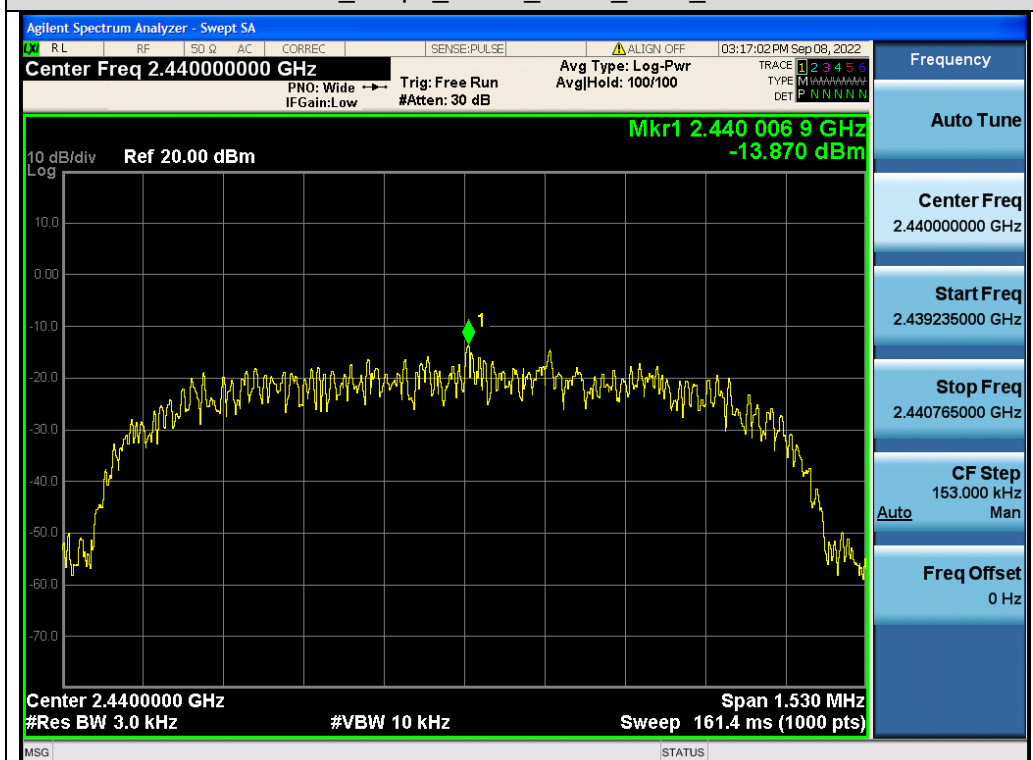
Test_Graph_GFSK_ANT1_2440_PSD
