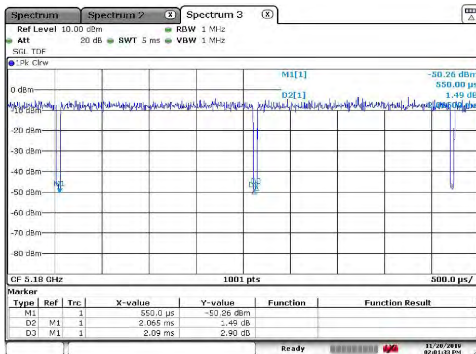
802.11a (SISO A)
