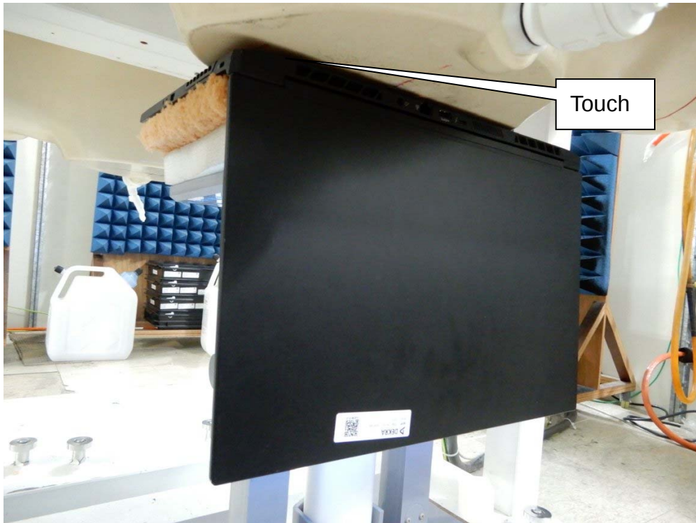
EUT Bottom-Aux
