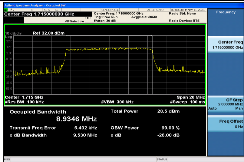
Band4-10MHz-QPSK-20000-50RB#0-8.9346
