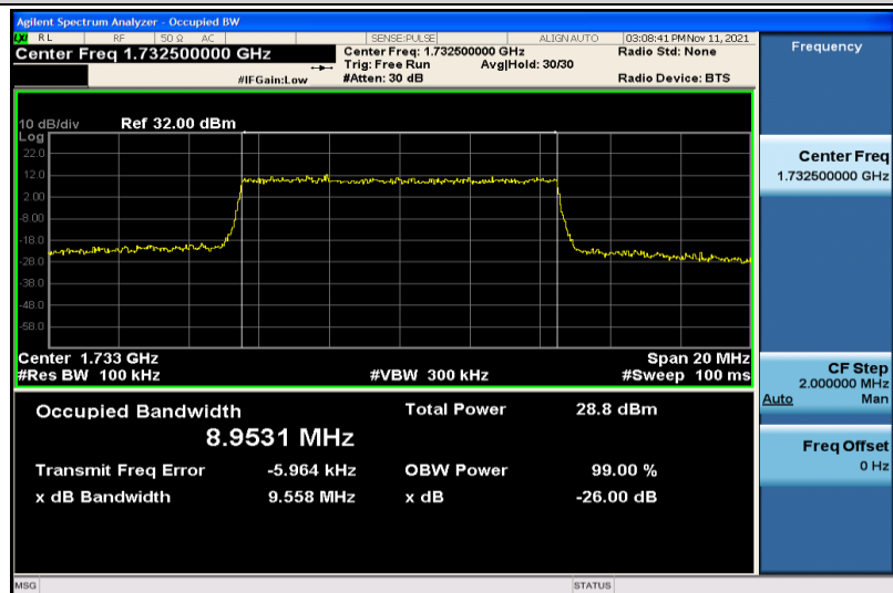
Band4-10MHz-QPSK-20175-50RB#0-8.9531
