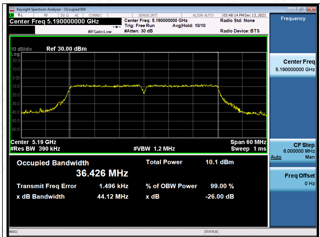
Test_Graph_802.11n40_ANT1_5190_MCS0_OBW
