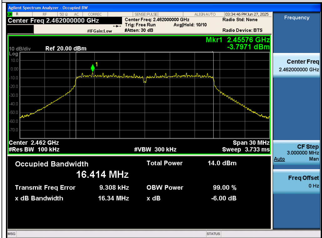
Test_Graph_802.11g_ANT1_2462_6Mbps_DTSSW
