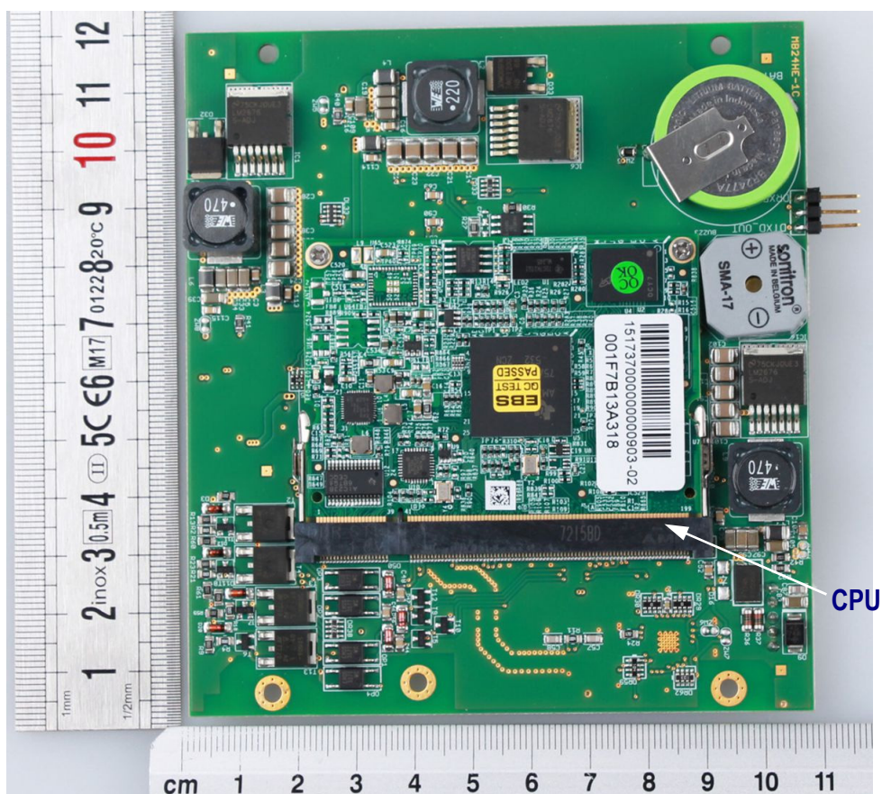
a). PCB: MB24HE
