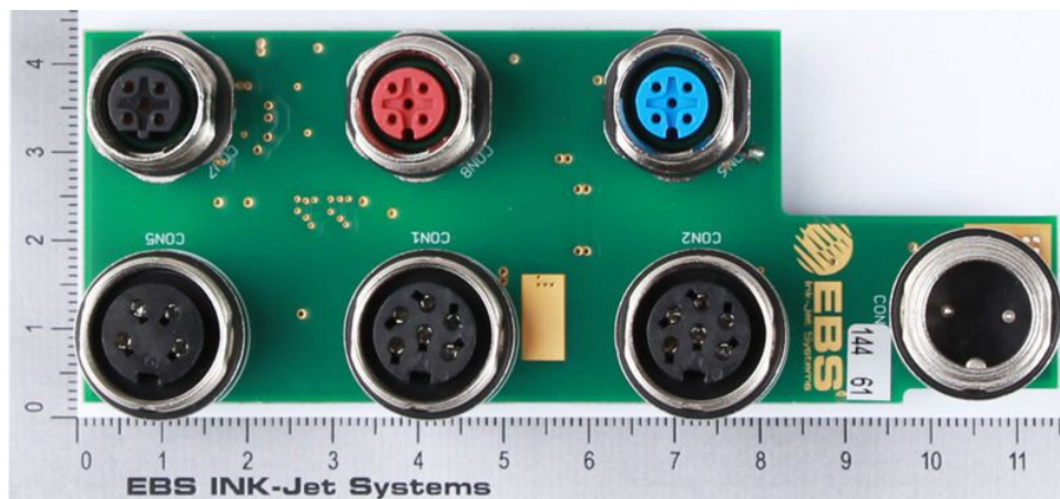
d). PCB: CN24HE
