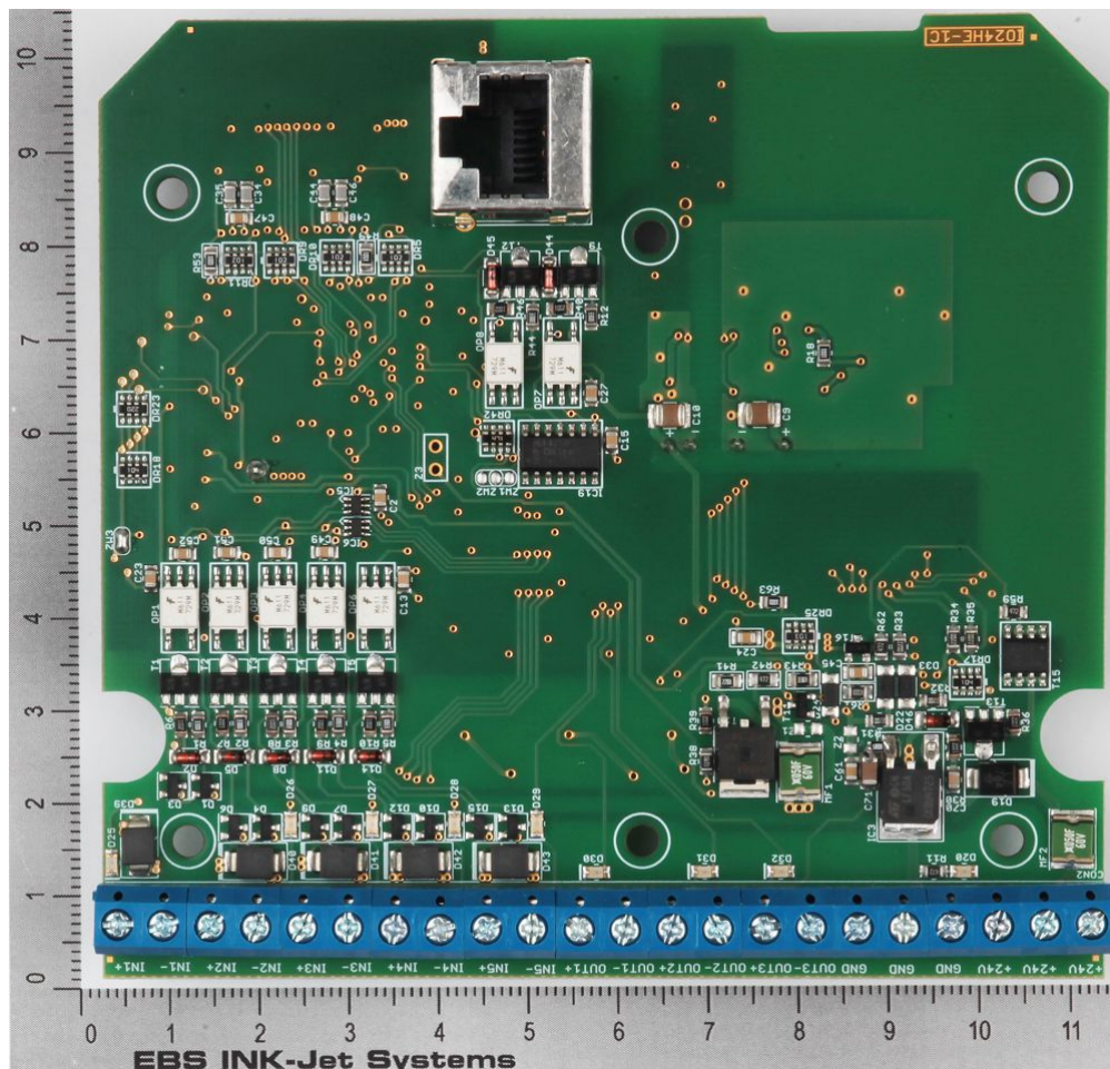
d). PCB: CN24HE
