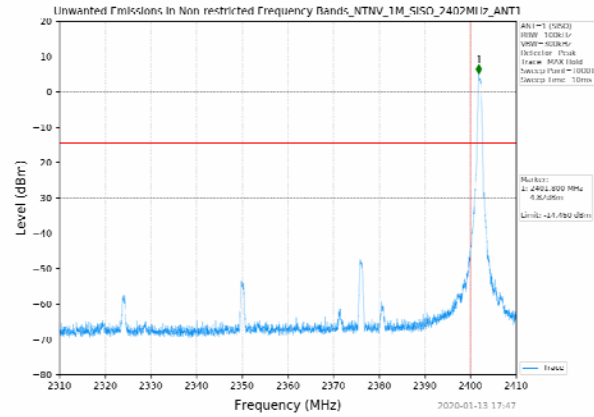
1M_2402MHz_SISO_ANT1
