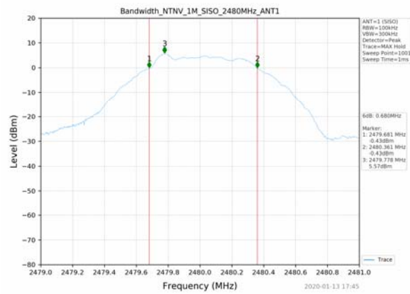
1M_2480MHz_SISO_ANT1
