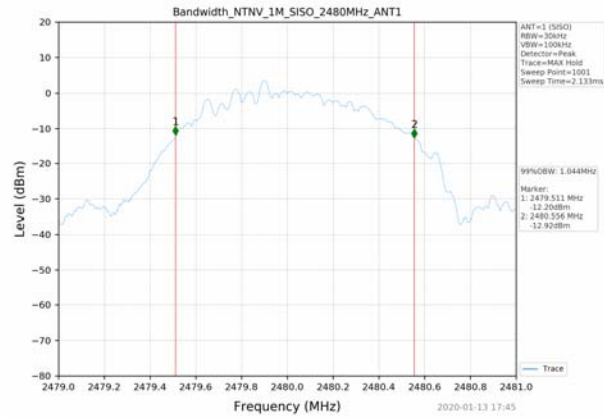
1M_2480MHz_SISO_ANT1
