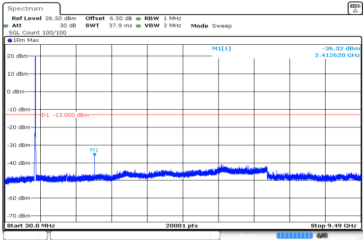
10MHz_Mid_QPSK_50@0 -36.32 dBm
