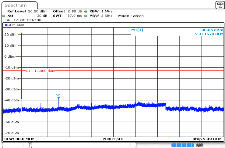
5MHz_Low_QPSK_25@0 -38.86 dBm
