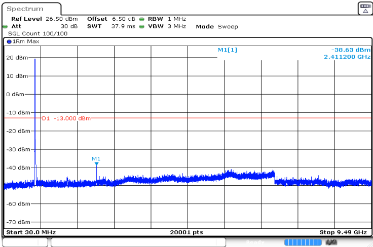
10MHz_Low_QPSK_50@0 -38.63 dBm
