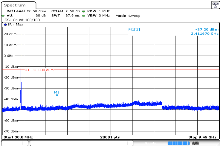
10MHz_High_QPSK_50@0 -37.29 dBm
