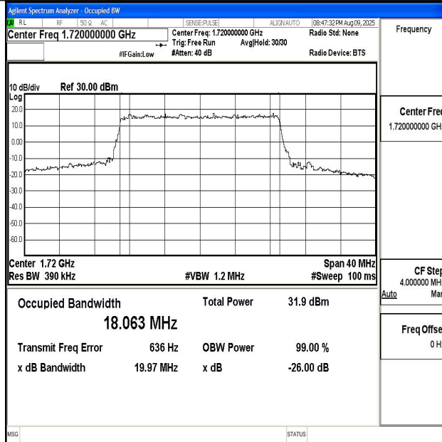
Band4-20MHz-QPSK-20050-100RB#0-PASS
