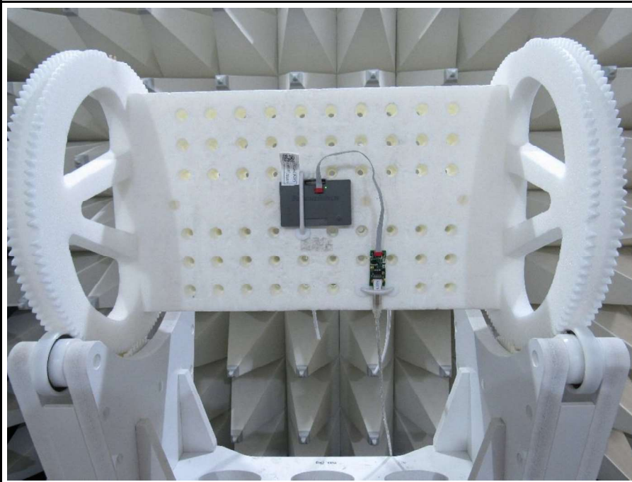
Setup EUT
