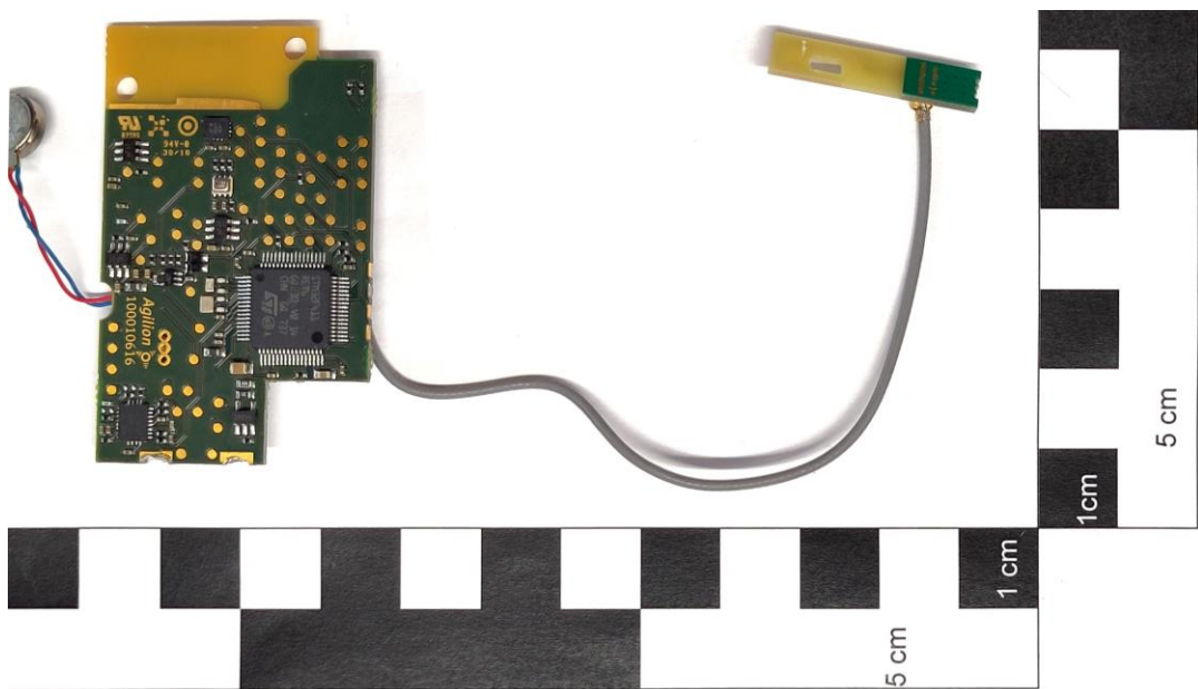
PCB Bottom
