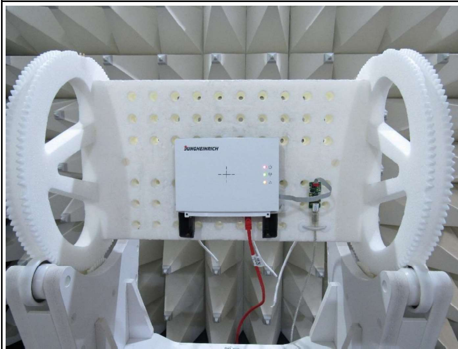
Setup EUT
