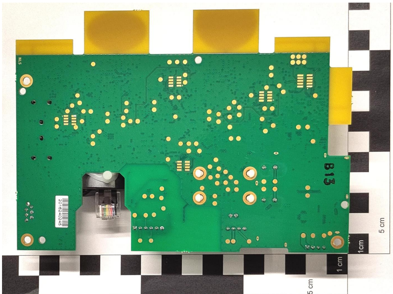
PCB Bottom
