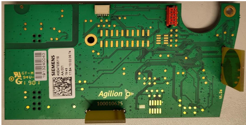
PCB Bottom
