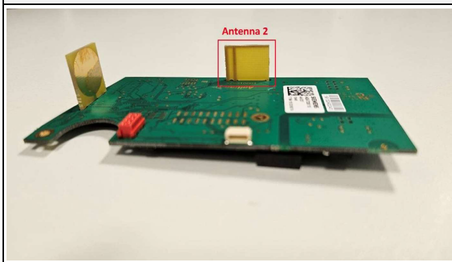
Antenna 2 - Bottom
