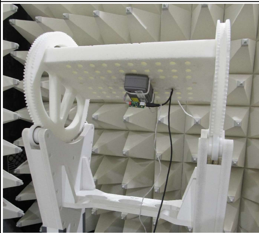
Setup EUT
