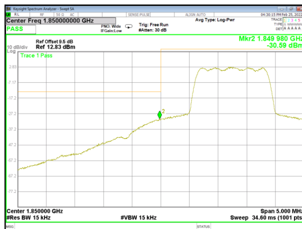
EVDO BC1 Low Band edge
