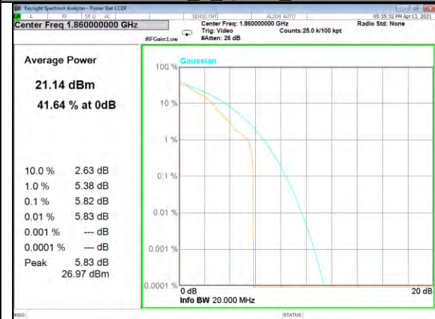
Band 2_1_Q16_Low
