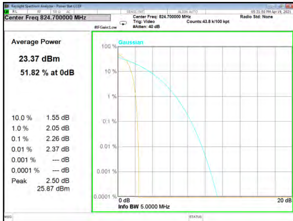
BC0_EVDO_Lower
