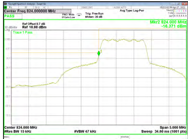
CDMA BC0 Low Band edge
