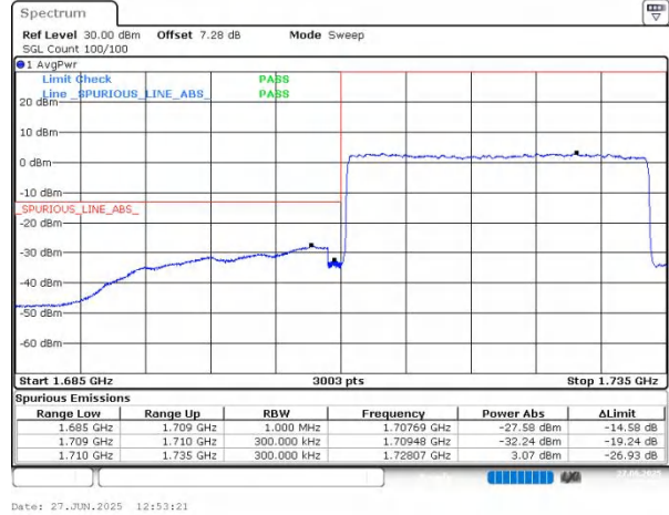
n66 SCS=15kHz DFT_QPSK BW=25MHz LowChannel=344500 RB=128@0
