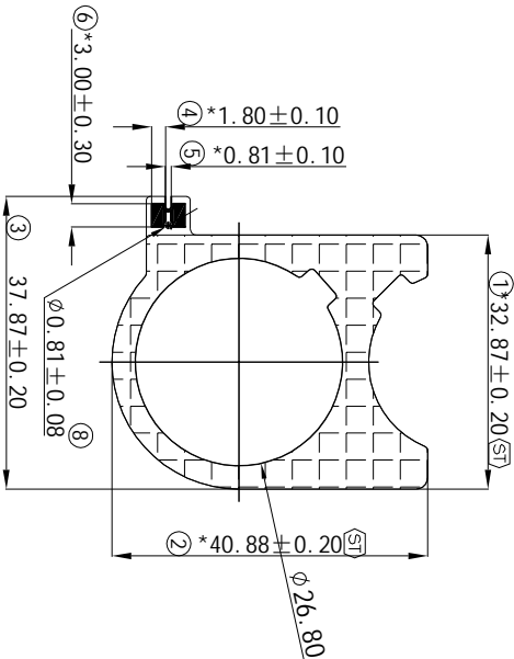
TOP (铁氧体面)
