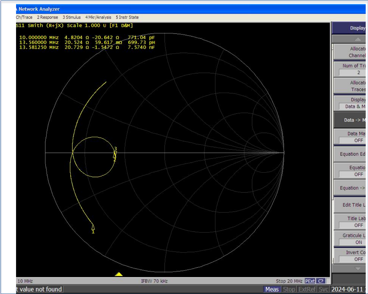
• 阻抗网分图
