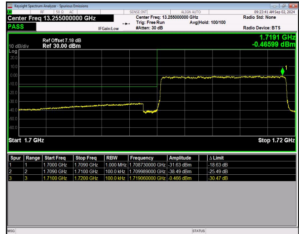
n66 SCS=15kHz DFT_256QAM BW=10MHz LowChannel=343000 RB=50@0 NVNT
