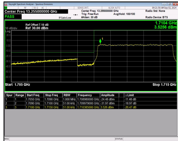
RB=25@0 NVNT
