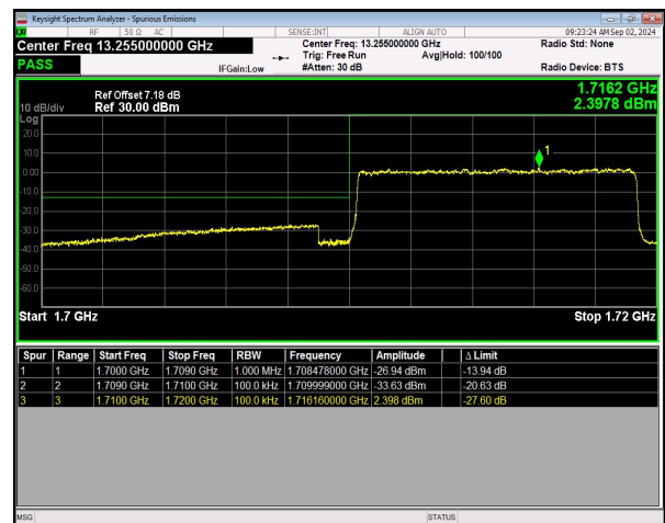
n66 SCS=15kHz DFT_16QAM BW=10MHz LowChannel=343000 RB=50@0 NVNT
