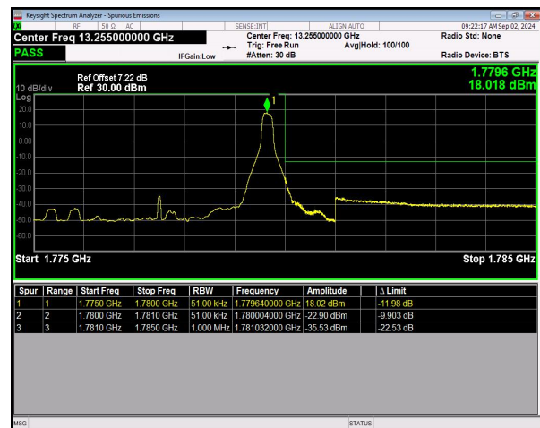
RB=1@24 NVNT
