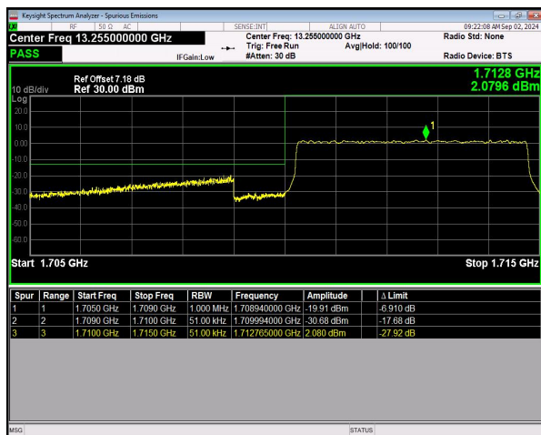
RB=25@0 NVNT
