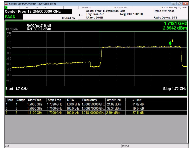
n66 SCS=15kHz DFT_QPSK BW=10MHz LowChannel=343000 RB=50@0 NVNT
