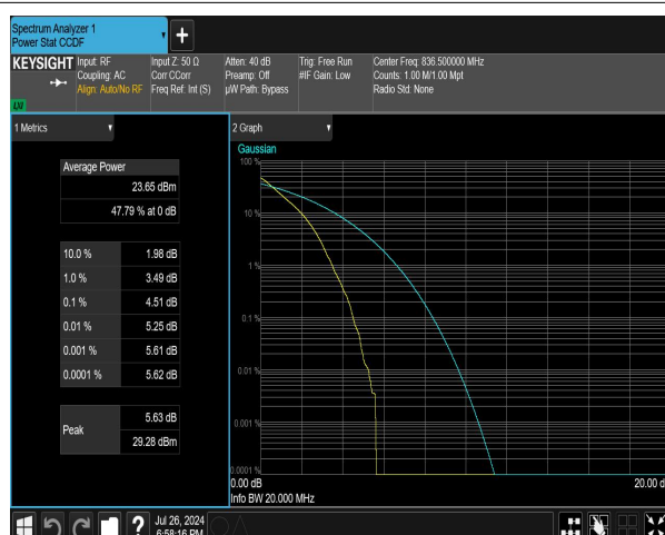
n5 SCS=15kHz DFT_BPSK BW=10MHz Channel=167300
