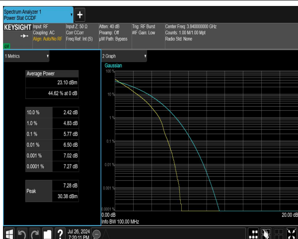
n77(3700-3980) SCS=30kHz DFT_QPSK BW=100MHz
