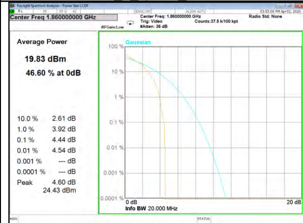
B25_1_Q16_Lower
