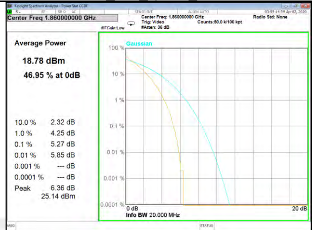
B25_100_Q16_Lower
