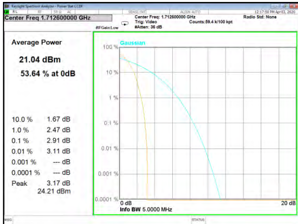
WCDMA B4_Lower
