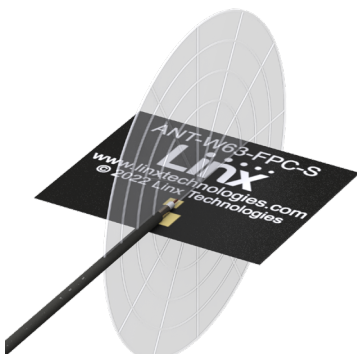
YZ-Plane Gain
