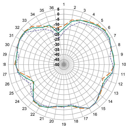
XZ-Plane Gain
