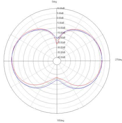
ZX-plane
