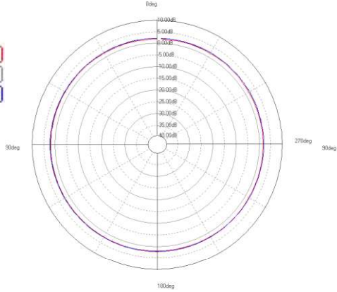
XY-plane
