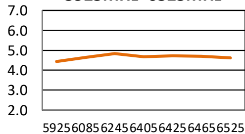
5925MHz~6525MHz
