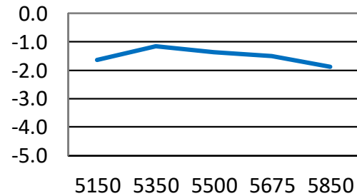
5150MHz~5850MHz
