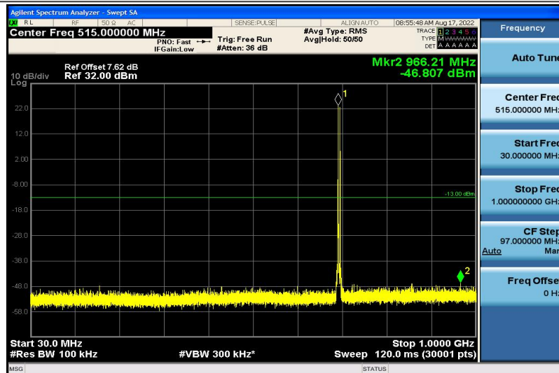
Band12-1.4MHz-QPSK-23017-1RB#0-30~1000MHz
