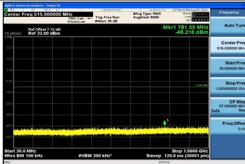
Band2-20MHz-QPSK-18700-1RB#0-30~1000MHz
