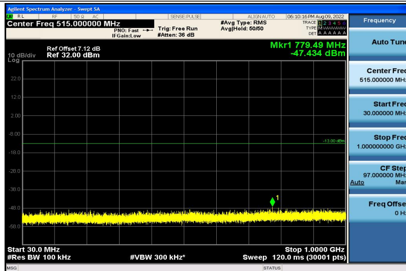
Band2-5MHz-QPSK-18625-1RB#0-30~1000MHz
