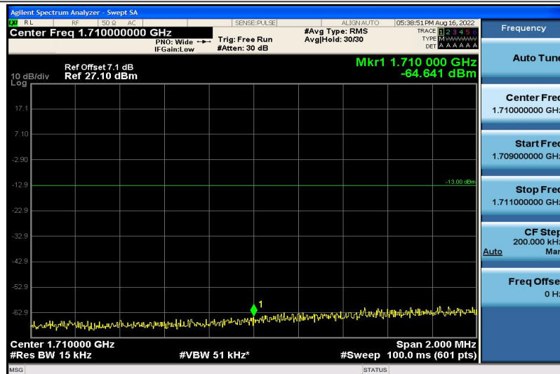
Band4-20MHz-QPSK-20050-1RB#5
