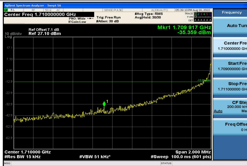
Band4-20MHz-QPSK-20050-6RB#0
