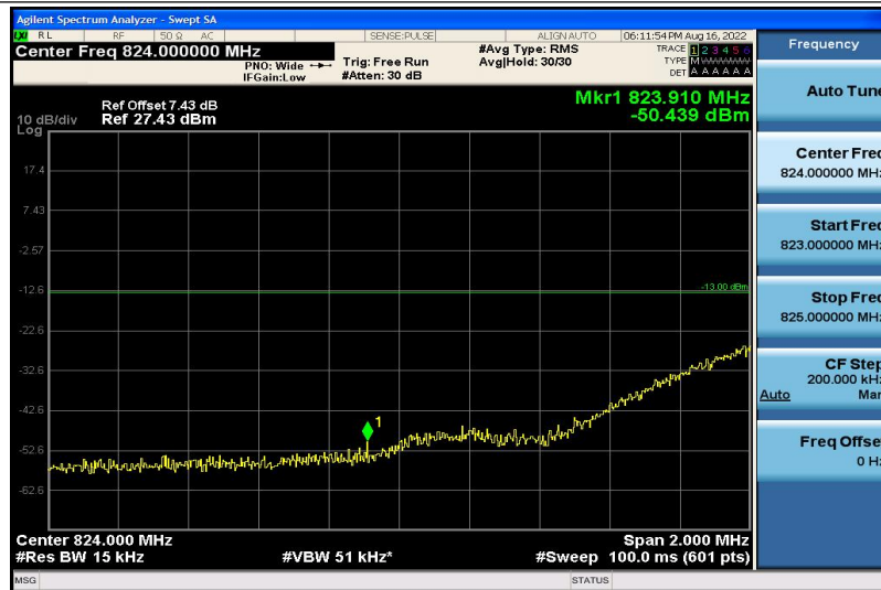
Band5-3MHz-QPSK-20415-1RB#5
