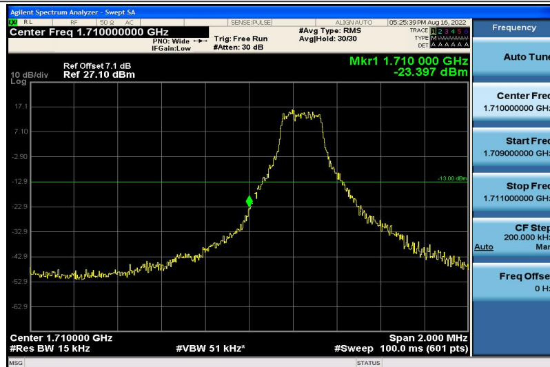
Band4-3MHz-QPSK-19965-1RB#0
