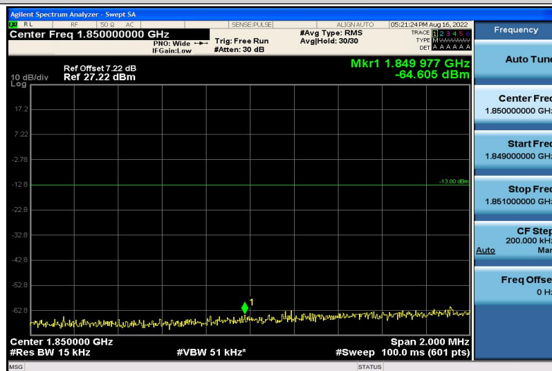
Band2-20MHz-QPSK-18700-1RB#5
