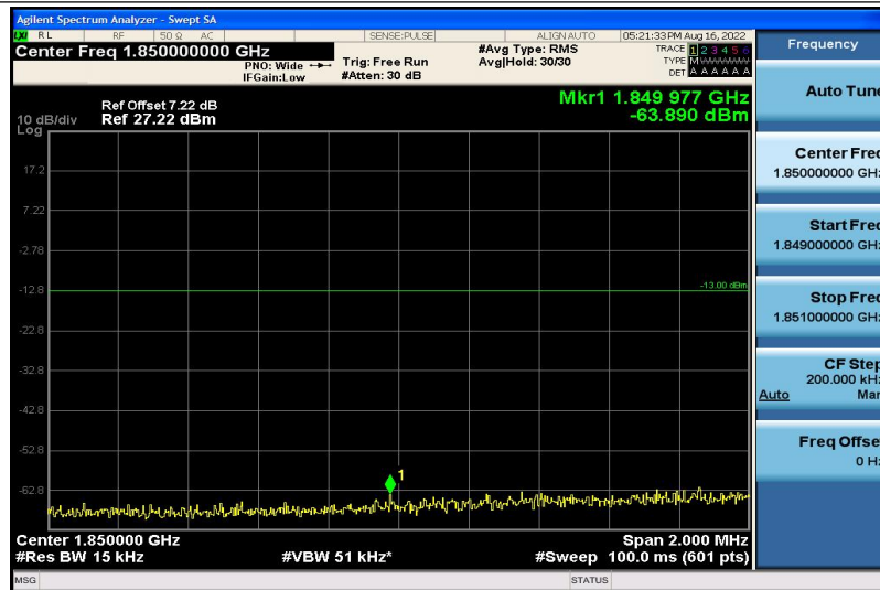
Band2-20MHz-16QAM-18700-1RB#5
