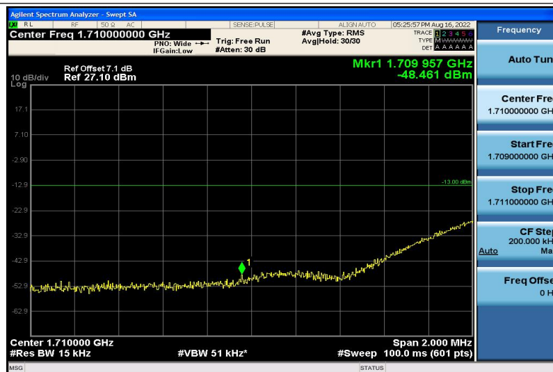
Band4-3MHz-QPSK-19965-1RB#5
