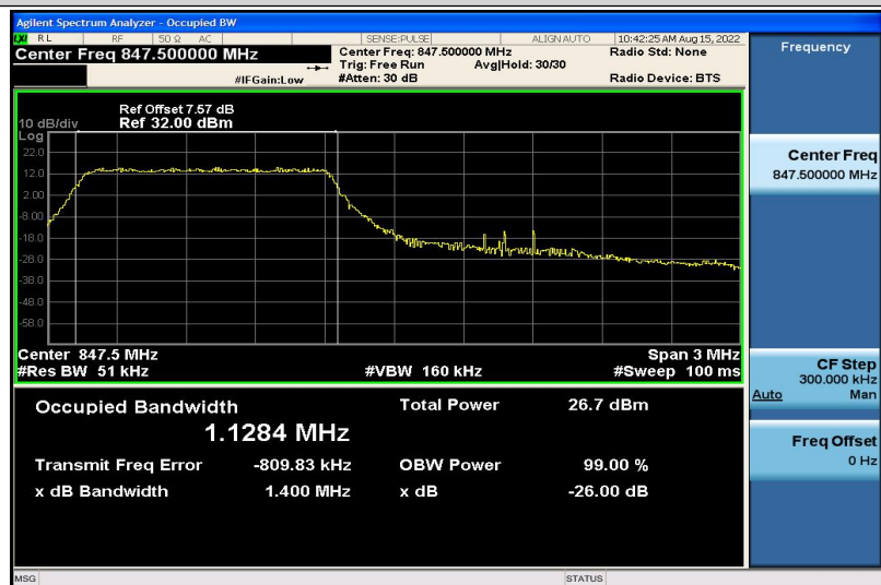
Band5-3MHz-QPSK-20635-6RB#0-1.1284
