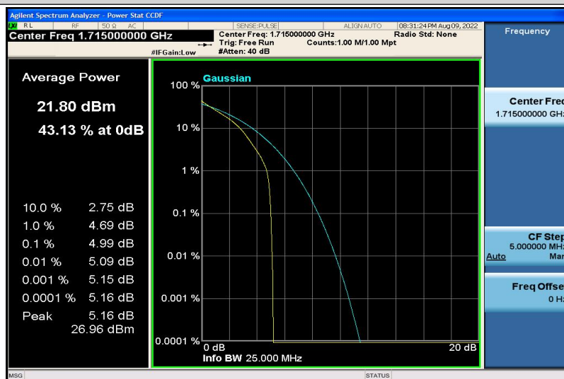
Band4-10MHz-QPSK-20000-6RB#0
