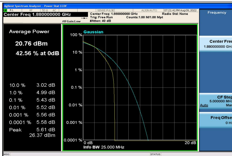
Band2-20MHz-16QAM-18900-6RB#0
