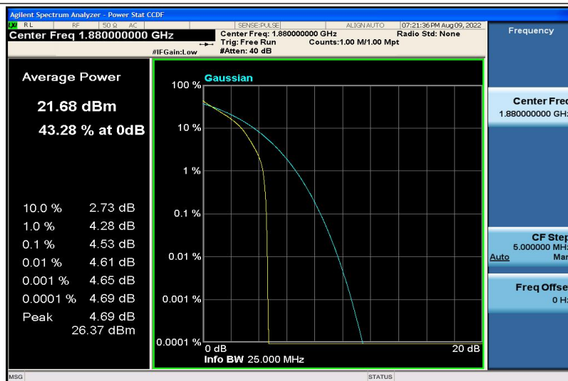
Band2-20MHz-QPSK-18900-6RB#0
