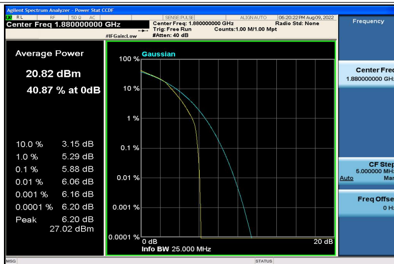
Band2-5MHz-16QAM-18900-6RB#0
