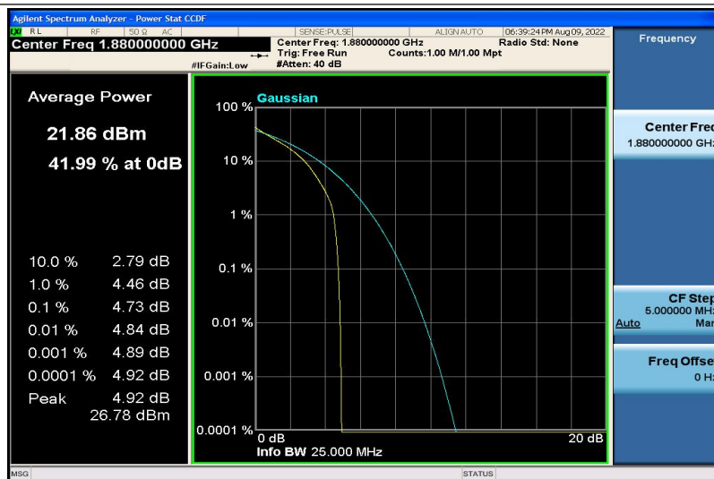
Band2-10MHz-QPSK-18900-6RB#0
