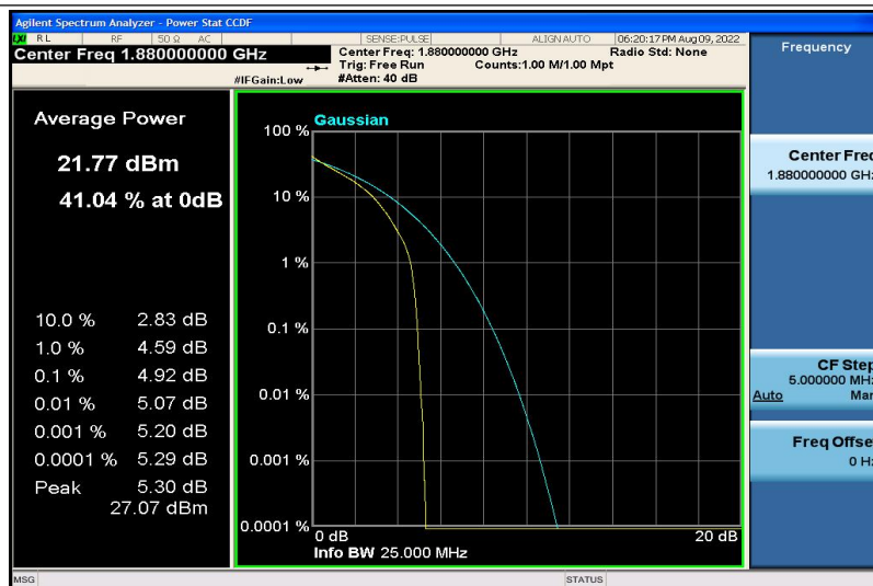
Band2-5MHz-QPSK-18900-6RB#0
