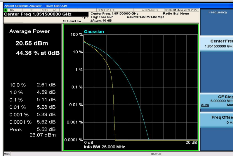
Band2-3MHz-QPSK-18615-6RB#0
