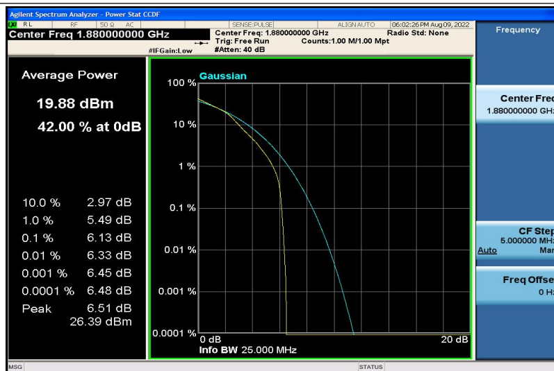
Band2-3MHz-16QAM-18900-6RB#0
