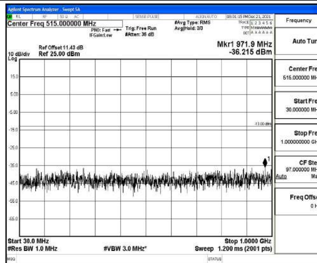
Band4-5MHz-QPSK-20175-1-0-Low-30-1000--36.22-PASS
