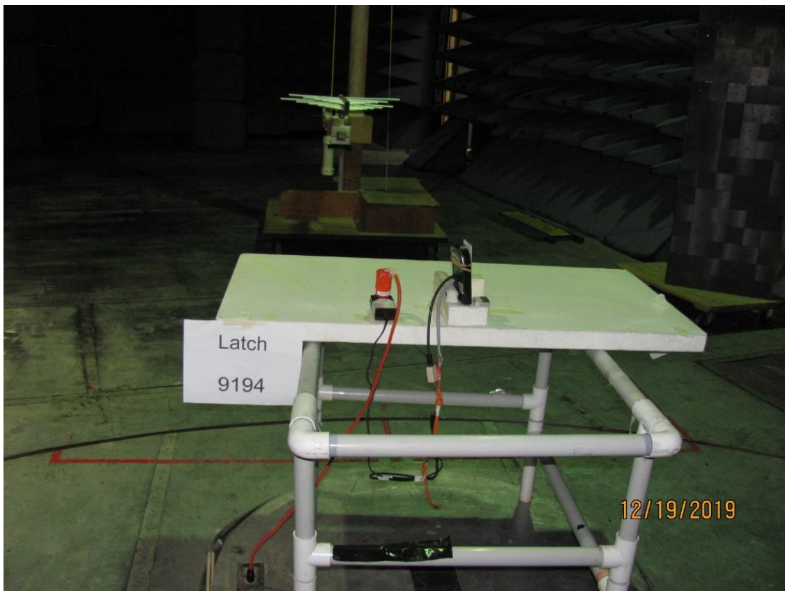
Log periodic Antenna
