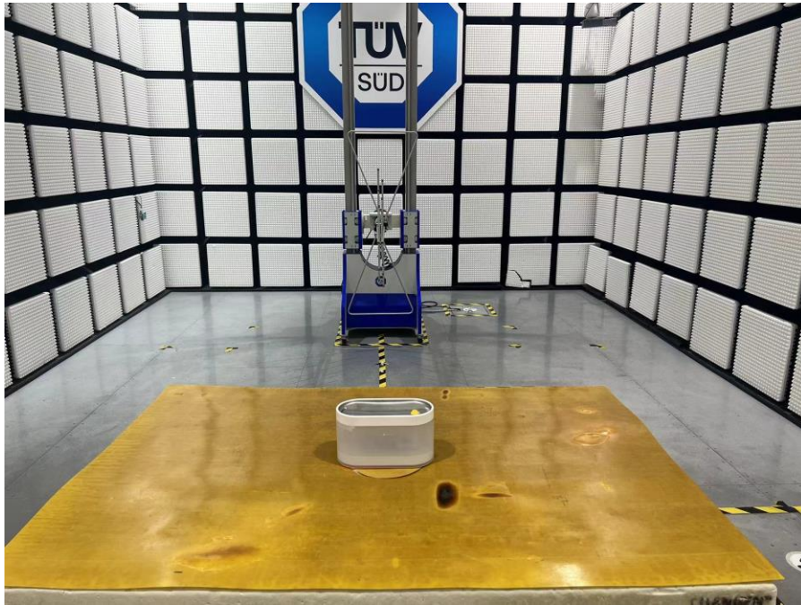
RSE 30-1000MHz
