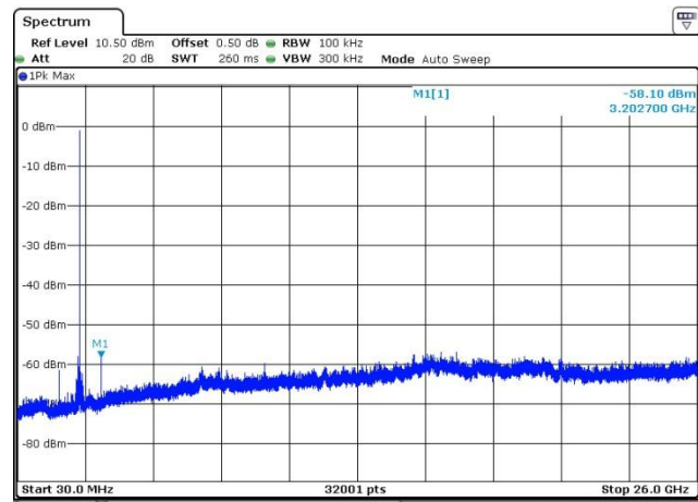
CH00-SE
