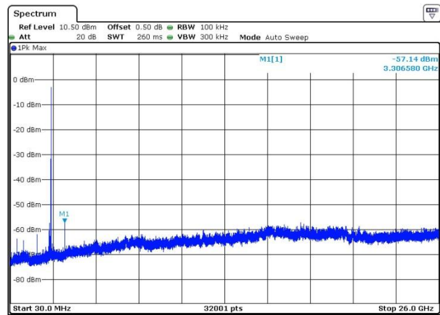
CH39-SE
