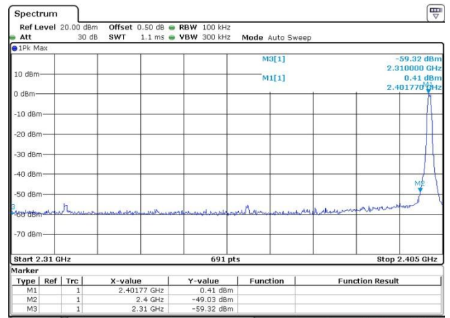
CH00-Bandedge
