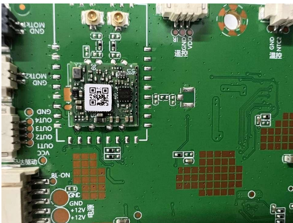
Photo 16 RF module
