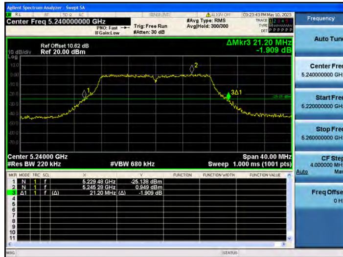
11A_Ant2_5240
