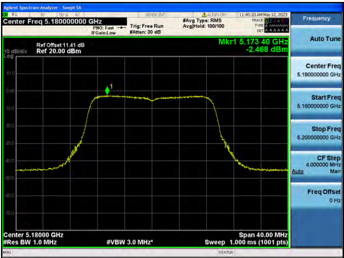
11AC20MIMO_Ant2_5180
