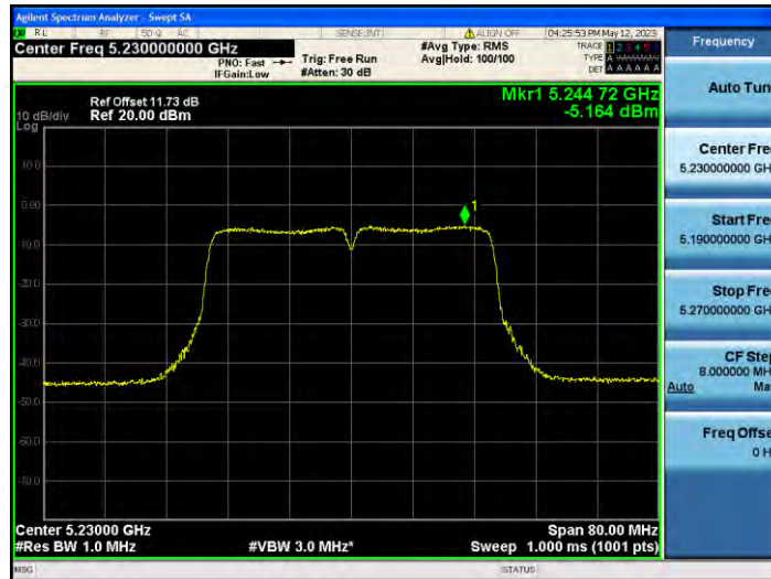
11AC40MIMO_Ant2_5230
