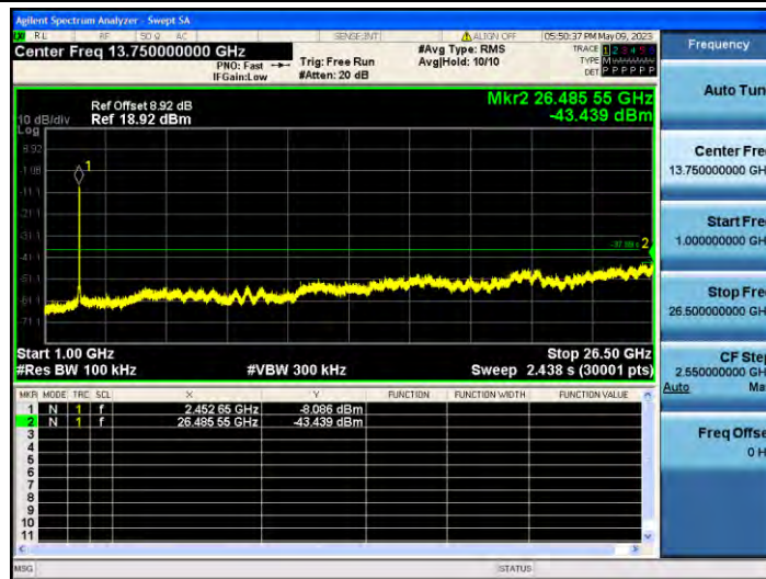
11N40MIMO_Ant2_2452_0~Reference
