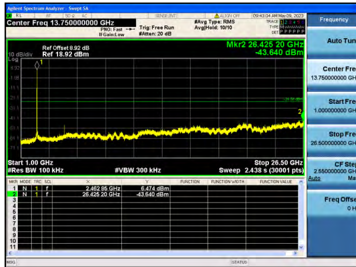
11B_Ant2_2462_0~Reference
