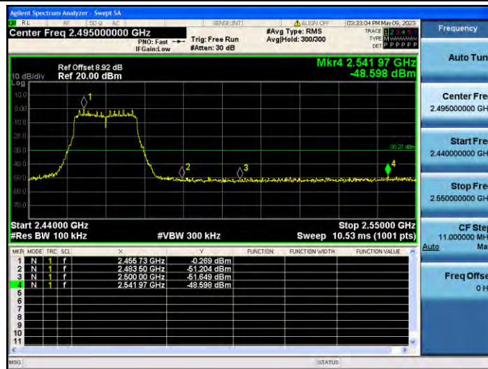
11N20MIMO_Ant2_High_2462
