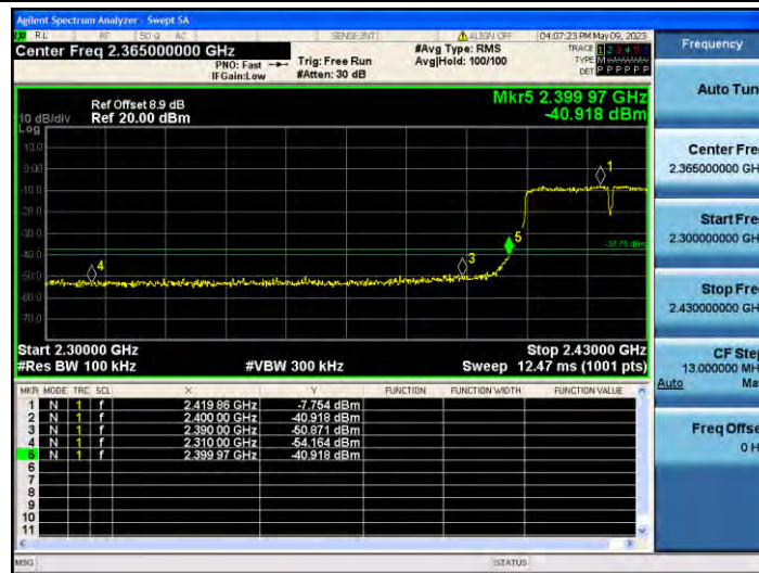
11N40MIMO_Ant2_Low_2422
