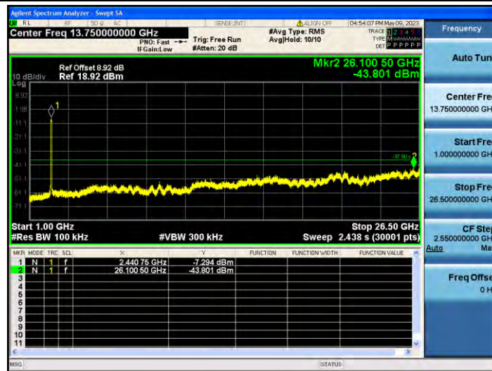
11N40MIMO_Ant2_2437_0~Reference
